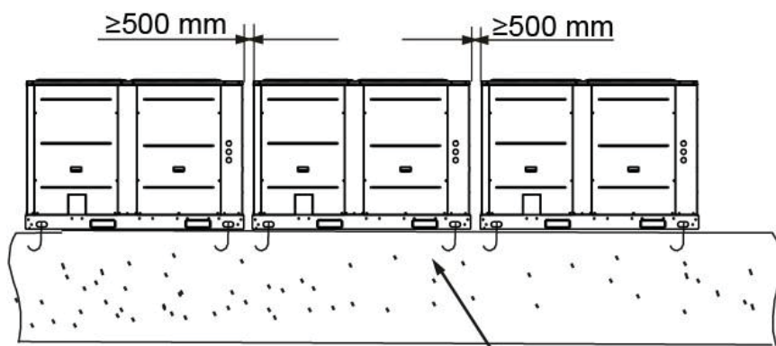
Фундаментные болты М12, 8шт на блок
