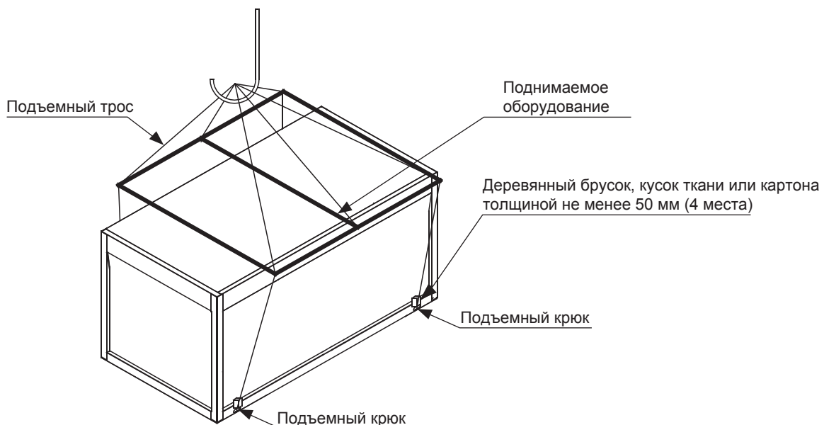
Рис. 2-1 Подъем агрегата
