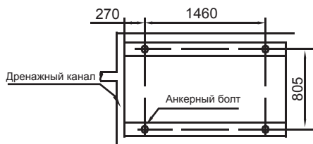
Схема с установочными размерами IMBL-F65A/NB
