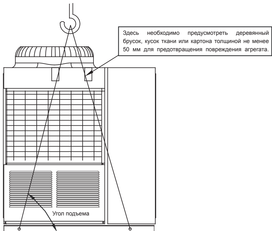
Рис. 2-1 Подъем агрегата
