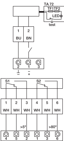
Схема 2 Серия 360
