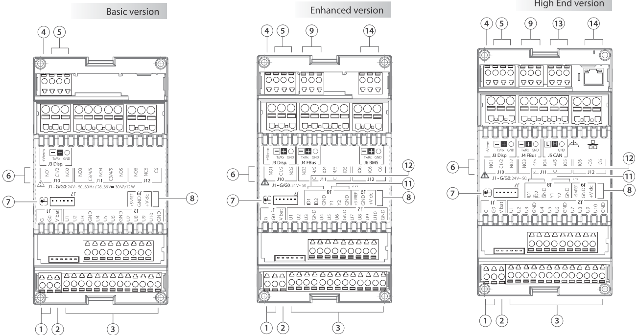
с.pCOmini - модель под врезной монтаж (вид сзади)
