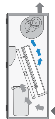
Восходящий поток, вытеснение сзади
