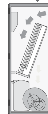
Нисходящий поток, вытеснение сверху
